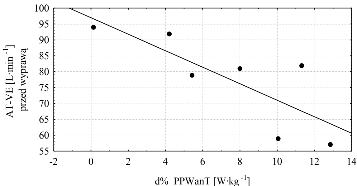
Rycina 17. Zależność procentu jaki stanowi zmiana maksymalnej mocy beztlenowej w stosunku do wartości sprzed hipoksji d\%_{PPWanT}[W \cdot kg^{-1}] a wartością progu przemian anaerobowych sprzed okresu hipoksji AT-VE [L \cdot min^{-1}] , r=-0,79 ; p=0,03 .
